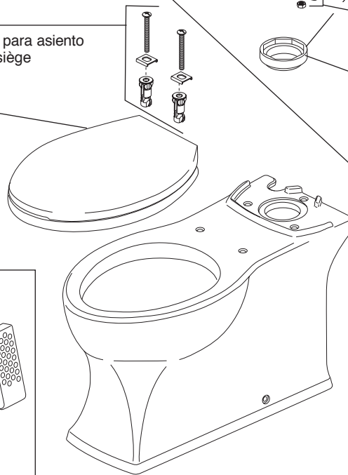
RP71200 Mounting Hardware Herraje para la instalación Pièces de montage
