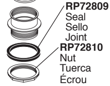
RP70878 Flush Valve Assembly Válvula de descarga Robinet de chasse
